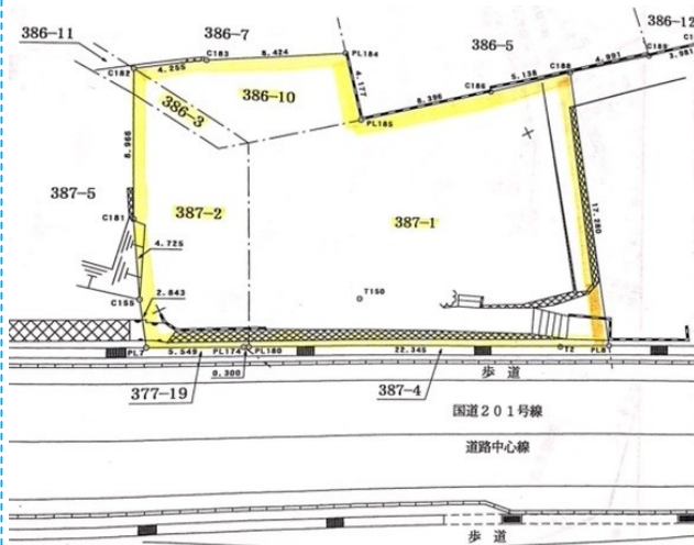
地積測量図
