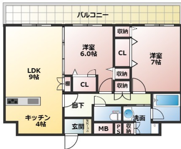
間取図
