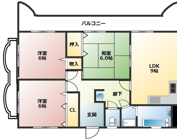
間取図
